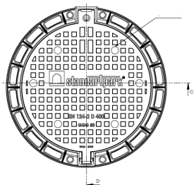
Vedere superioara
