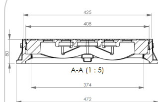
secțiune laterală
