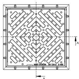
Secțiune superioară
