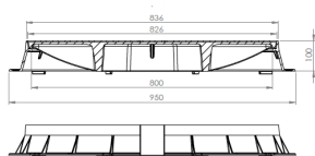
Schita vedere laterala
