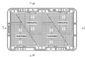
Sectiune superioara
