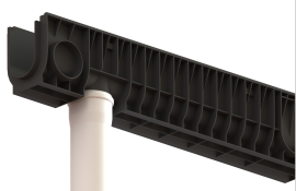
Conexiune verticală
