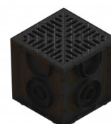
Kit camin PP EASY patrat Negru echipat cos parafrunzar si gratar PP A15 250x250 (0867081)
