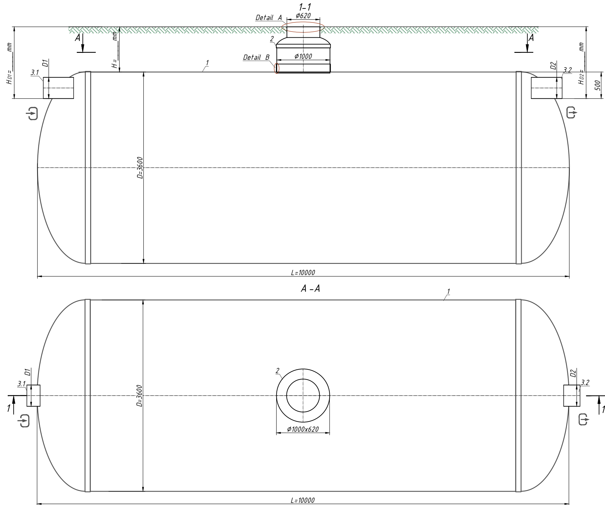
A -Manhole design*
