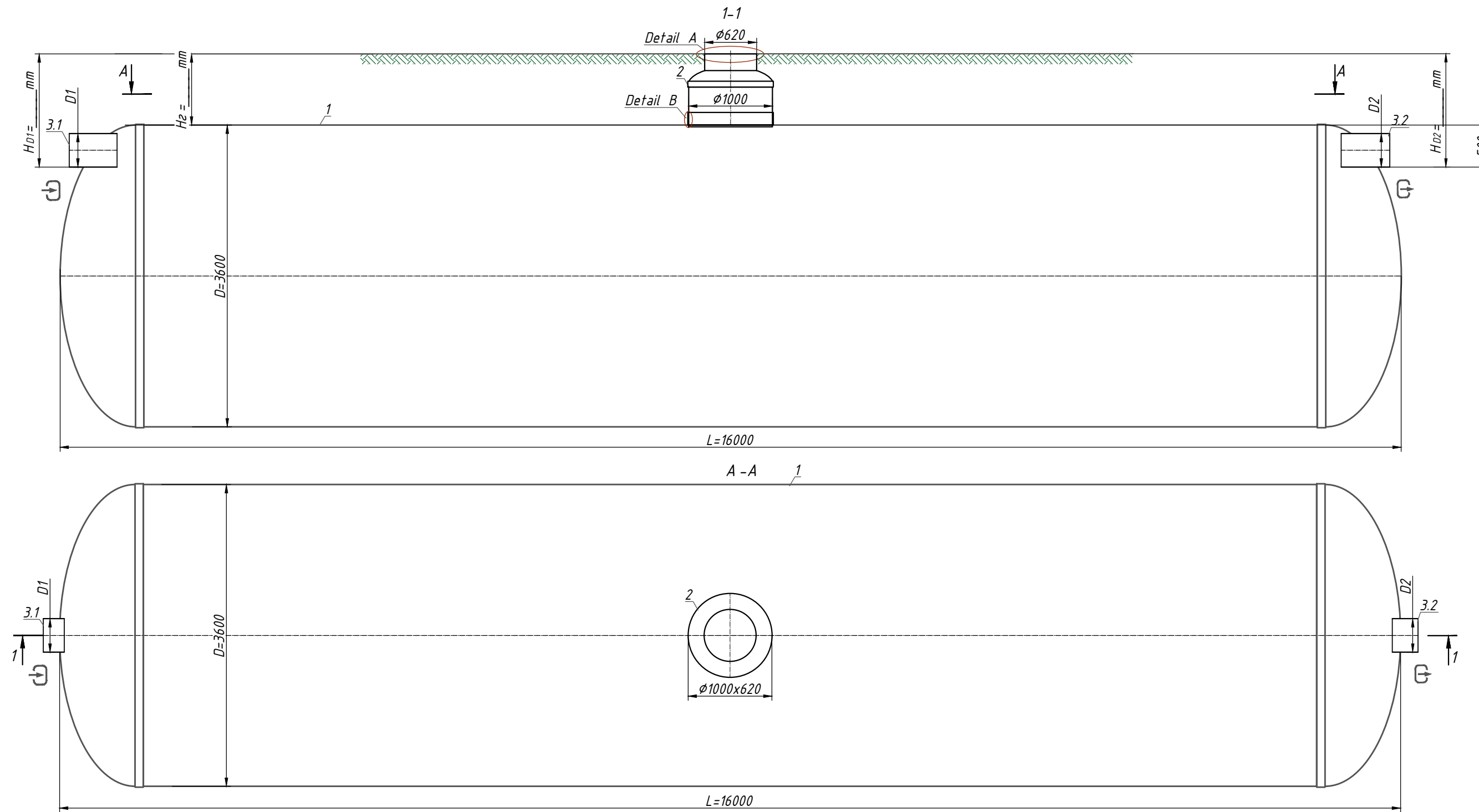
A -Manhole design*
